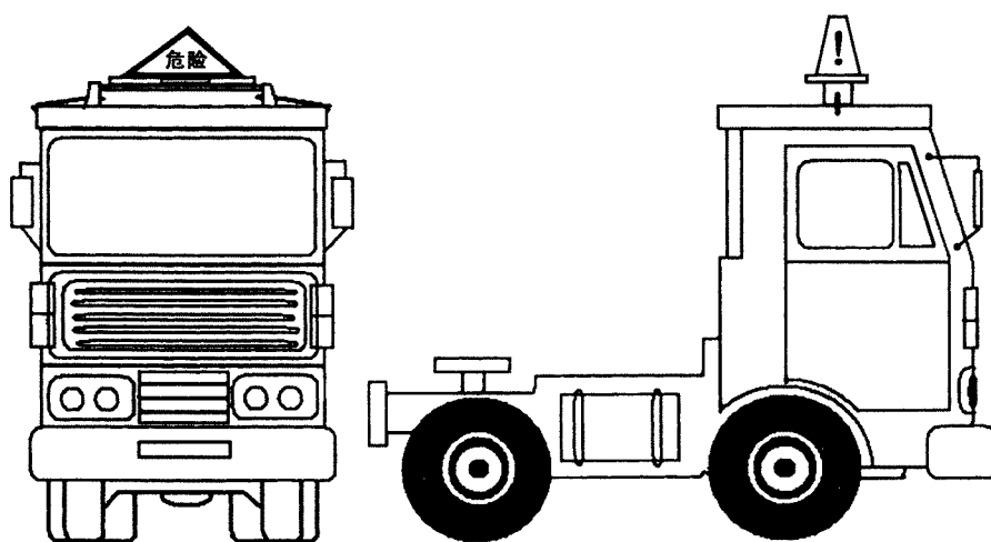
图 B.2 B 型标志灯安装位置
