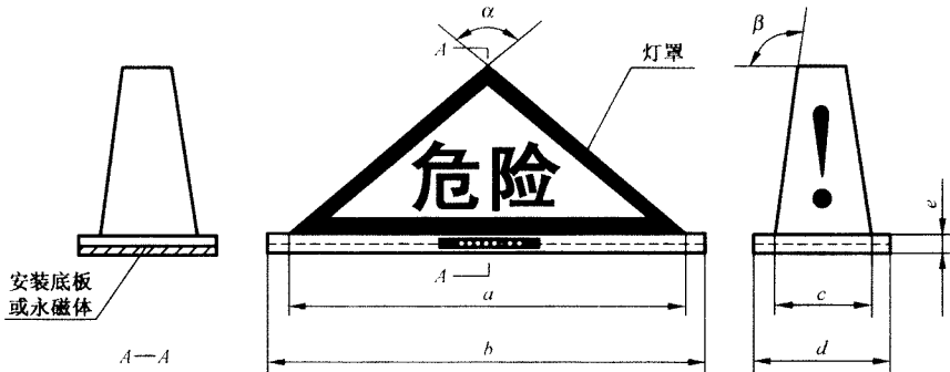
图 1 A 型标志灯
