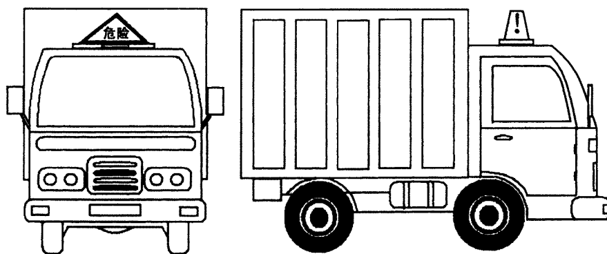
图 B.1 A 型标志灯安装位置
