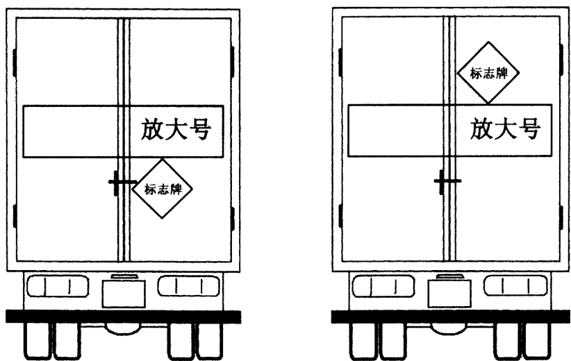
图 C.2 厢式车辆标志牌悬挂位置
