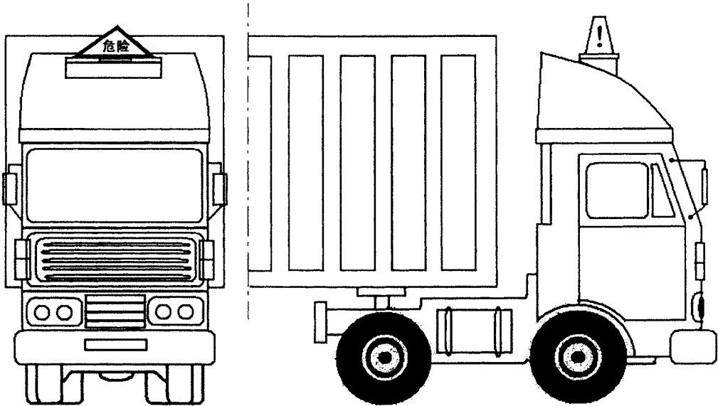
图 B.3 C 型标志灯安装位置
