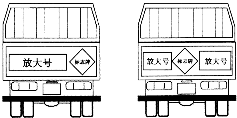
图 C.1 低栏板式车辆标志牌悬挂位置
