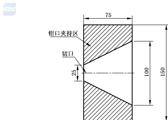
图 1 梯形法撕裂强力试样夹持示意图
