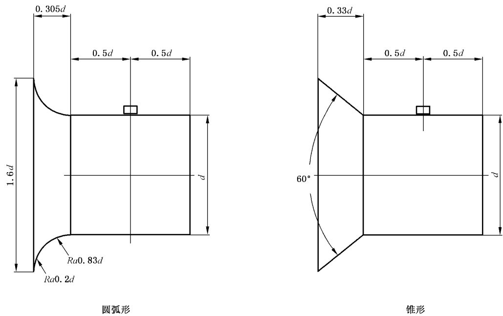
图 4 集流器外形尺寸
