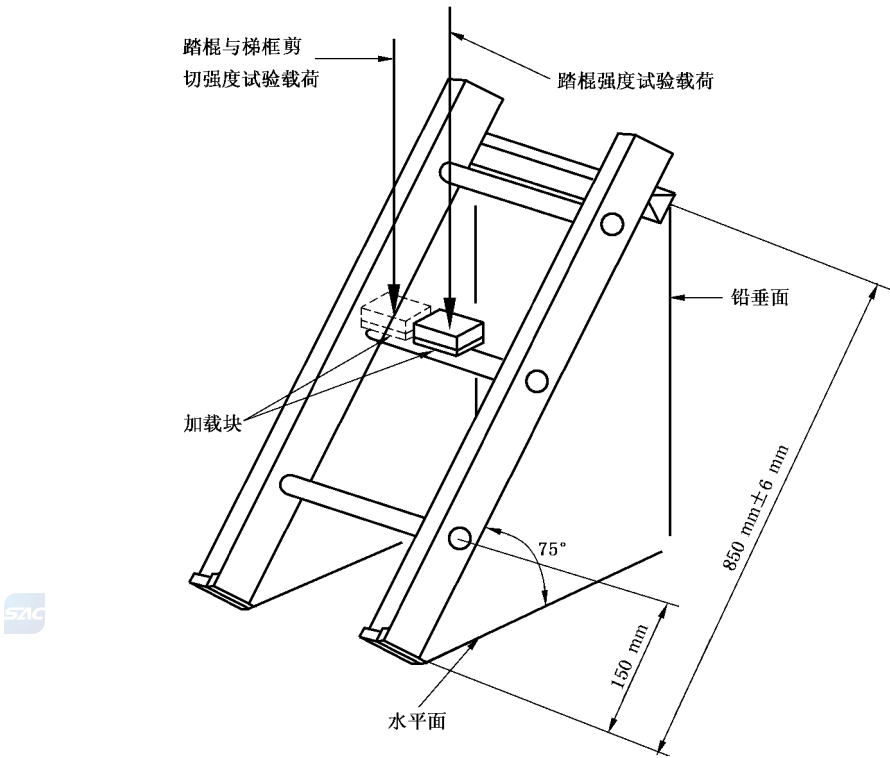
图 5 踏棍强度试验和踏棍与梯框剪切强度试验示意图
