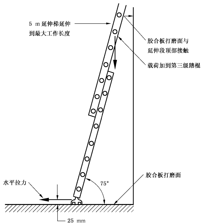
图 11 梯脚滑动试验示意图
