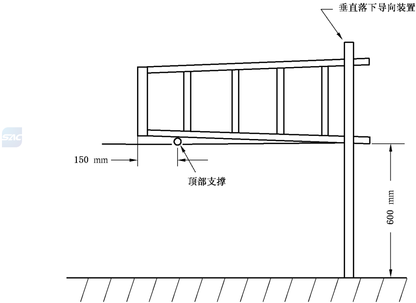
图 17 前后梯框悬臂落下试验示意图
