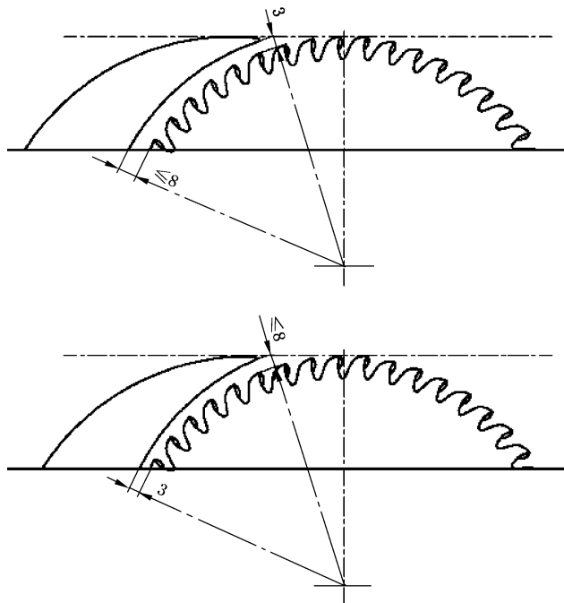
图 3 分料刀的定位极限
