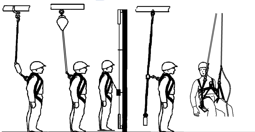
图 A.3 坠落悬挂安全带示意图
