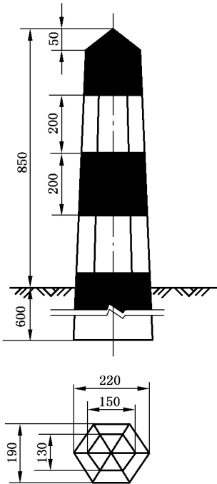
图 16 道口护桩
