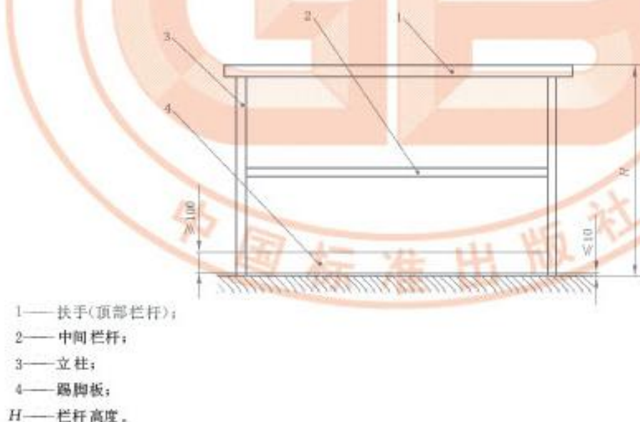
图1 防护栏杆示意图
