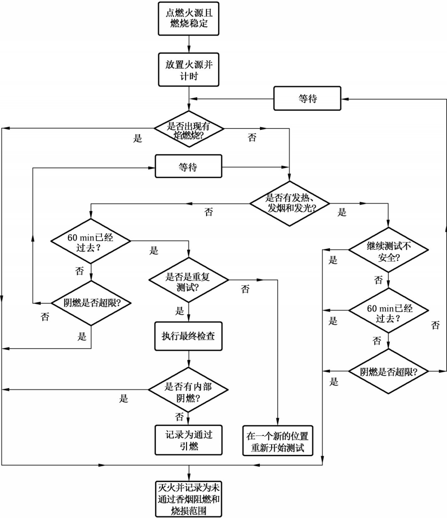
图 A.1 香烟引燃试验流程图
