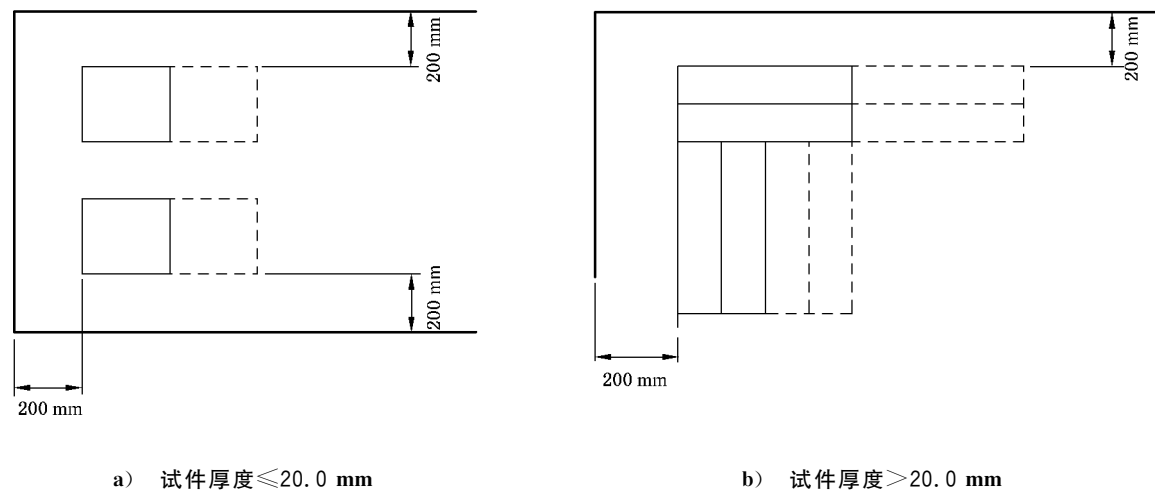
图 2 抗弯强度试件截取位置
