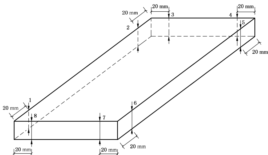
图 1 厚度测量位置
