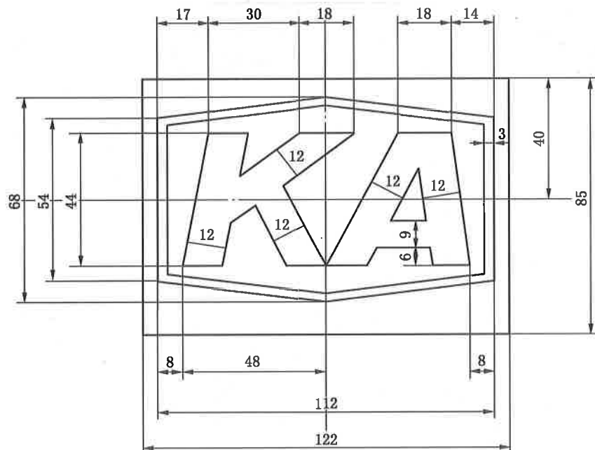
图 3 煤矿矿用产品安全标志标识图形及参数
