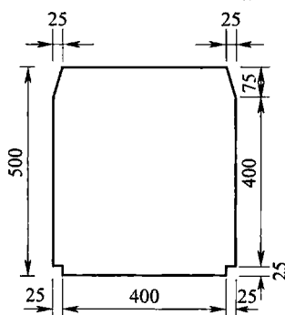
图 13 车行横通道的断面建筑限界(cm)
