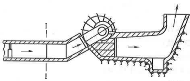
图 3 离心式通风机测压断面位置图
