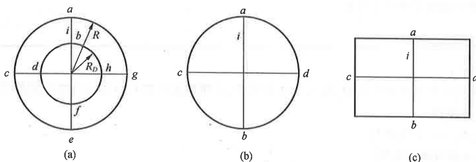
图 1 静压测点安设位置示意图
