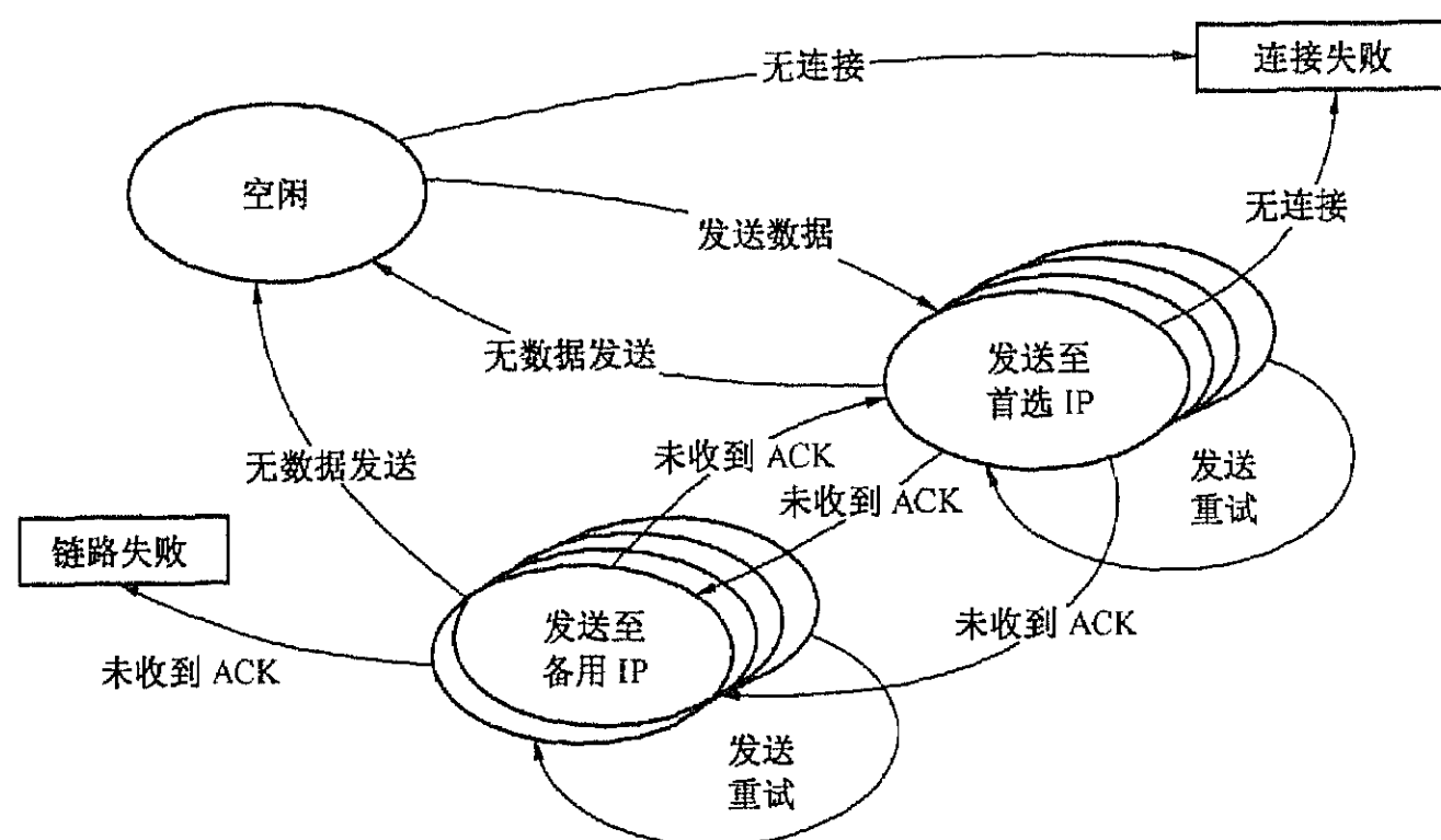
图 3 UDP/IP 数据报的发送
