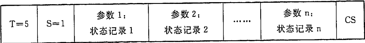
图 A. 12 历史状态记录消息数据的结构
