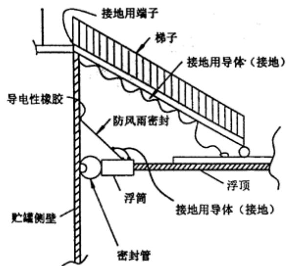
图 7 浮顶与储罐本体跨接
