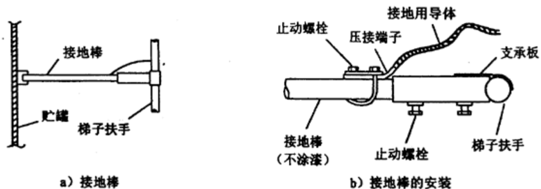
图 9 用接地棒消除静电
