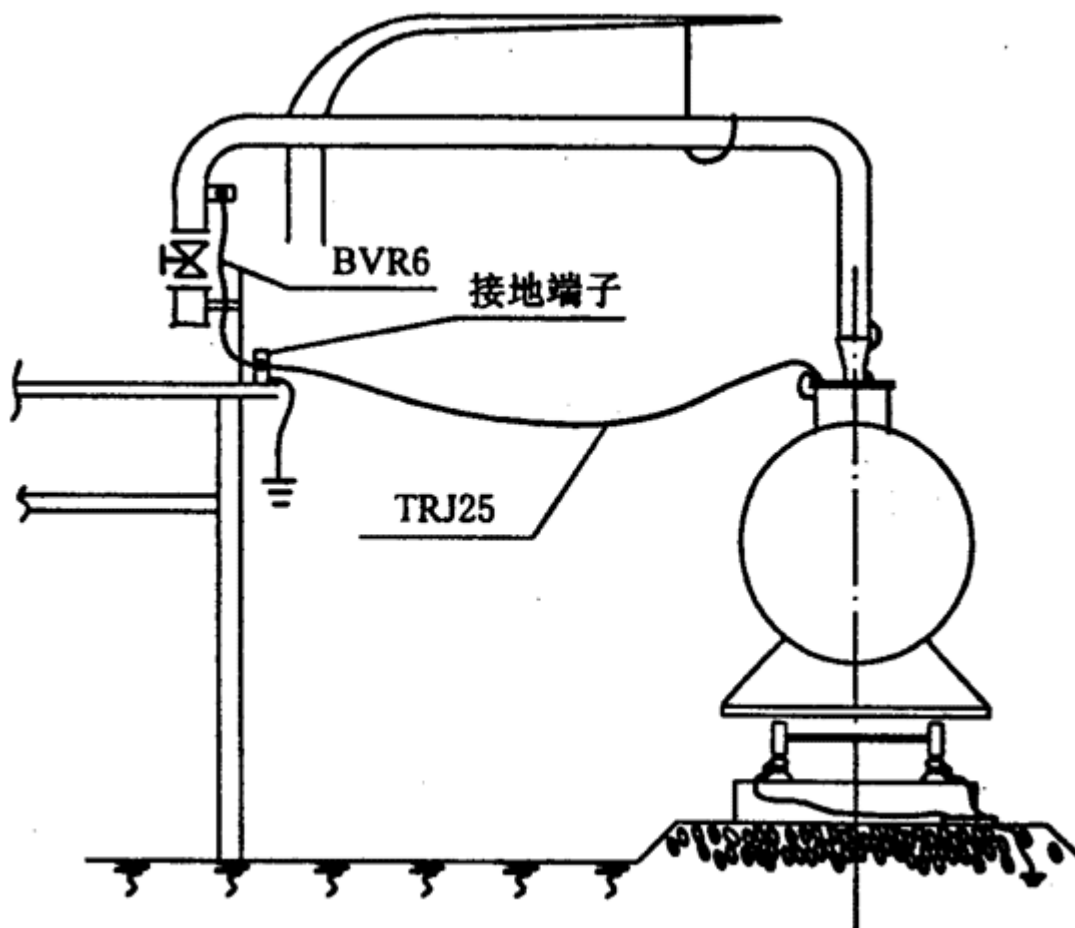
图 15 火车槽车接地示意
