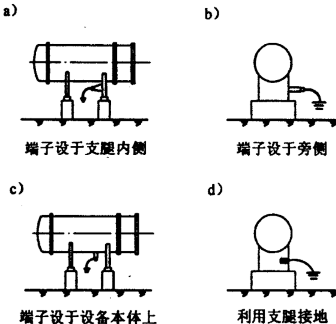
图 4 固定设备接地端子位置
