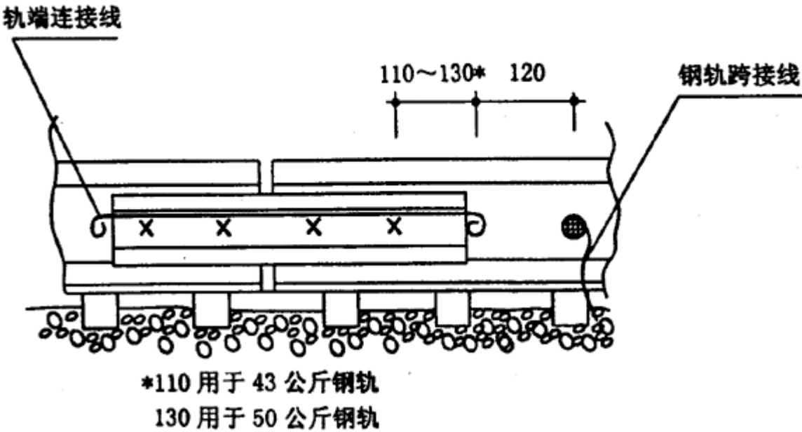
图 13 轨端跨接示意图
