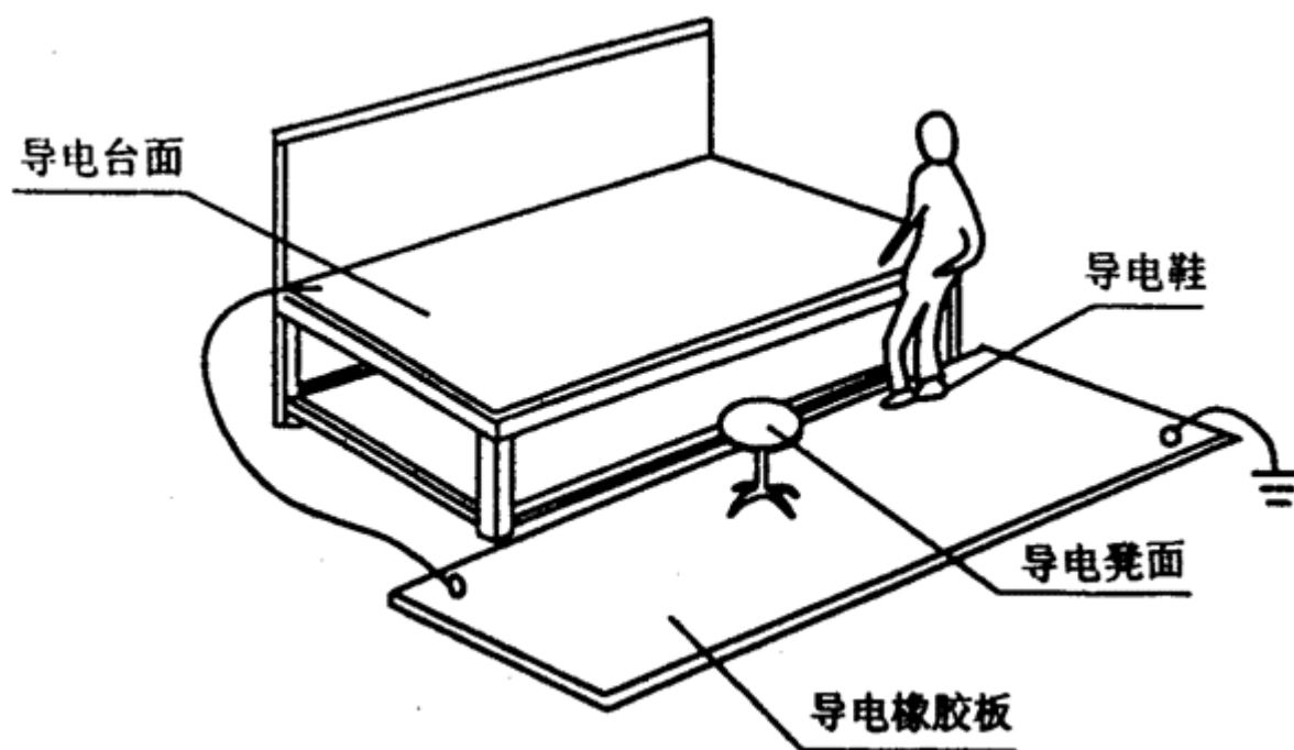
图 17 人体静电接地环境示意
