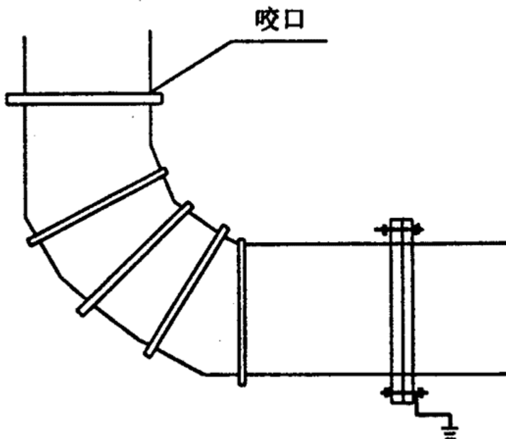
图 11 风管、保温层罩连接
