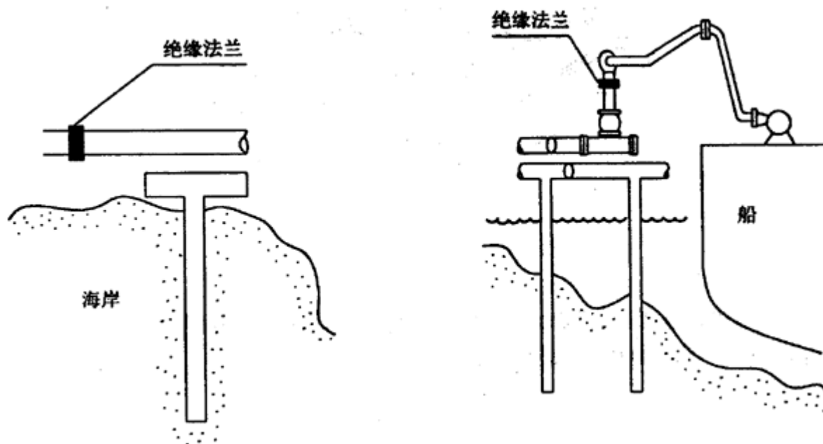
图 16 绝缘法兰使用示意
