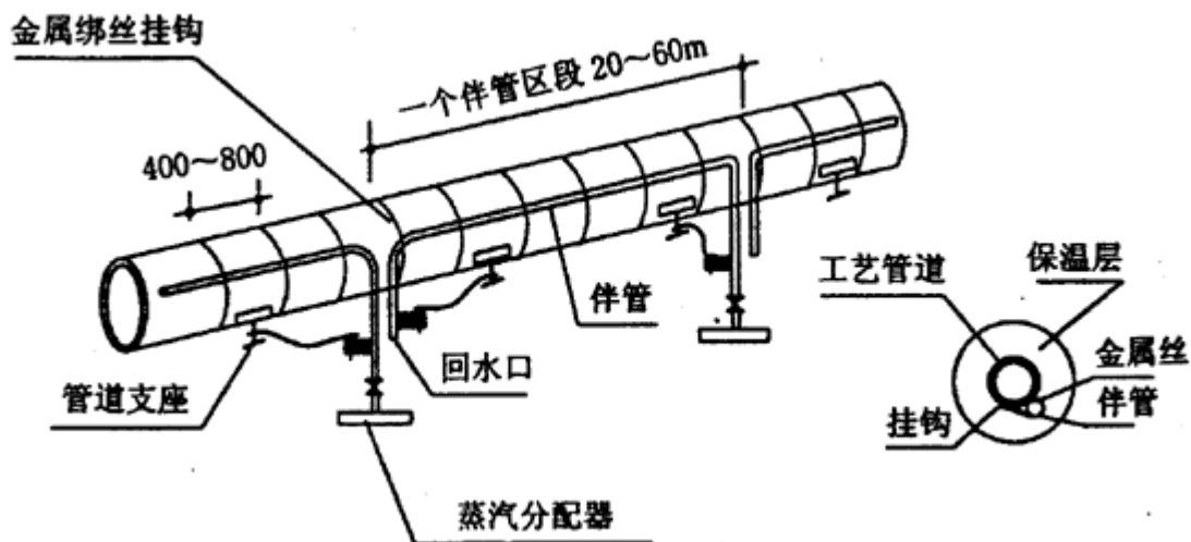
图 10 蒸气伴管与工艺管道连接示意
