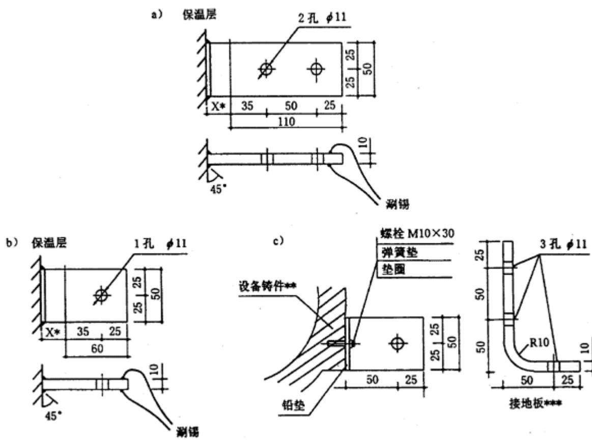
图 3 专用接地板组装示意图
