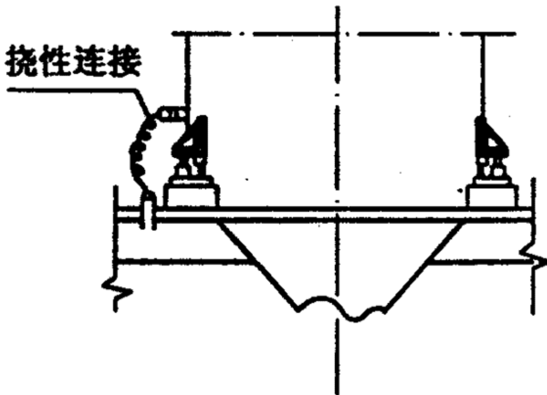
图 5 振动设备接地方案
