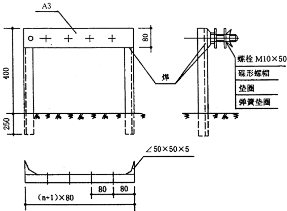
图 2 框架式接地端子排板
