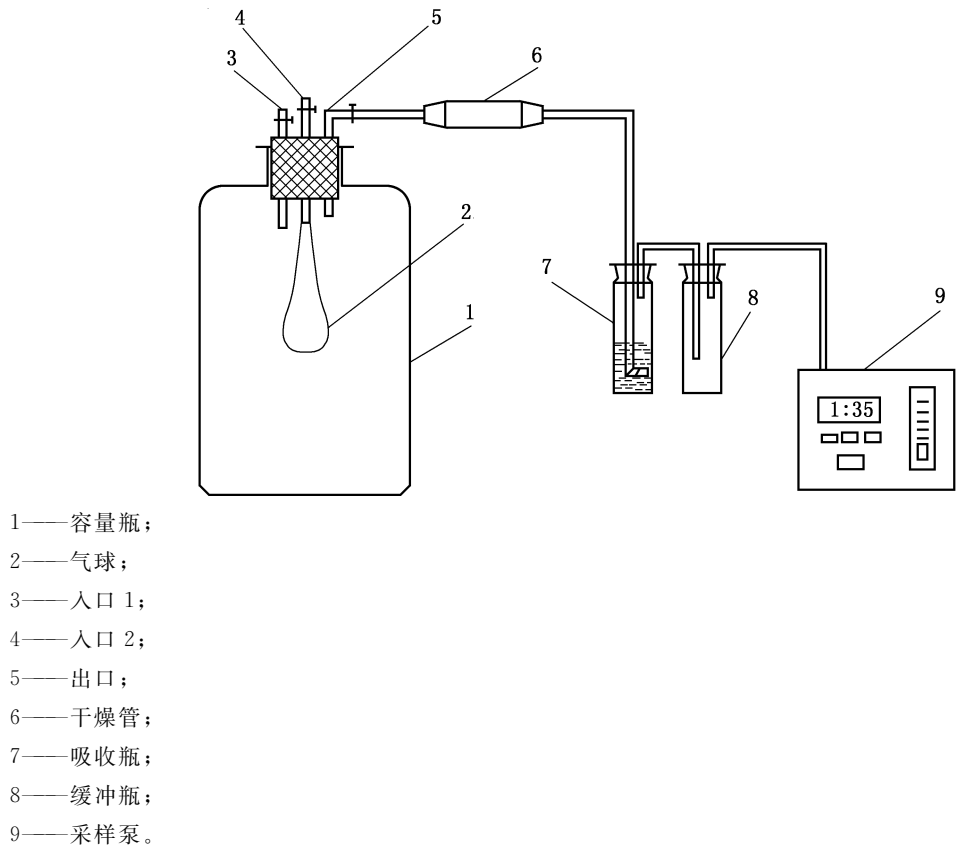
图 A.2 采样系统示意图
