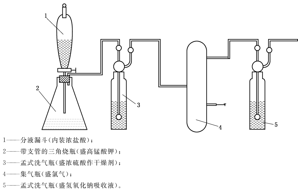
图 A.1 氯气制备系统示意图
