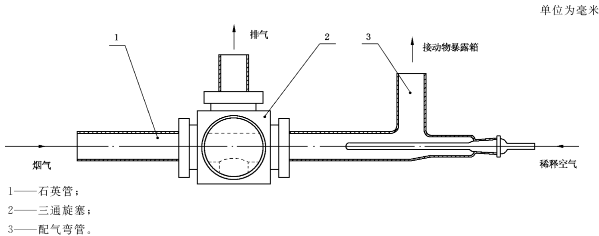
图 4 烟气采集配给组件
