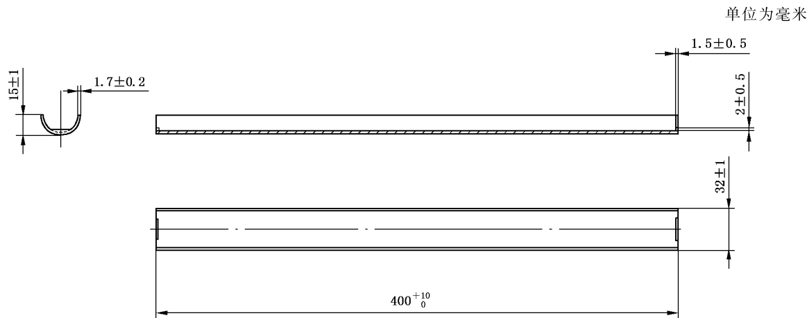
图 3 石英试样舟
