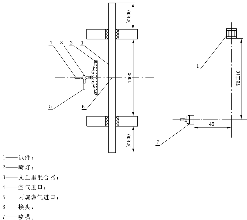
图 A.2 喷灯和试件的布置
